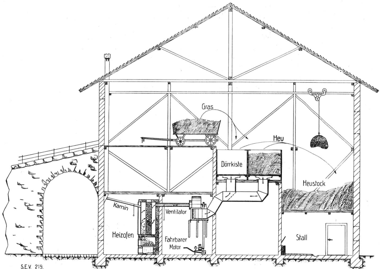
Fig. 1. Schema einer Grasdörnanlage.
