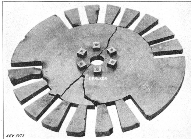
Fig. 5. Zersprungene Versuchsscheibe aus einem defekten Rotorkörper.
