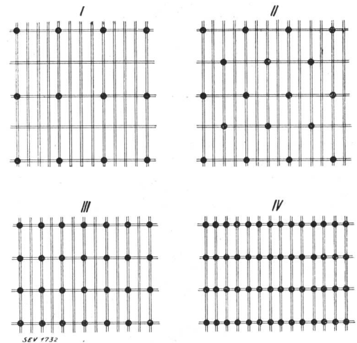
Fig. 5. Anordnung der Verteiltransformatoren für verschiedene Belastungsdichten. Die Linien bedeuten Verteiler 120/208 V (beidseitig der Strassen), die Punkte Transformatorstationen 500 kVA.
