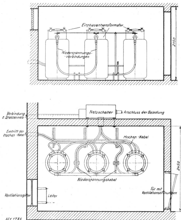
Fig. 9. Typische Transformatorstation im Innern eines Gebäudes.
