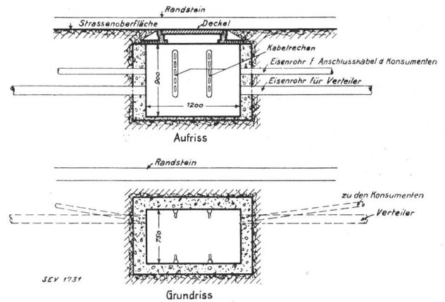
Fig. 4. Typischer Anschlusskasten.
