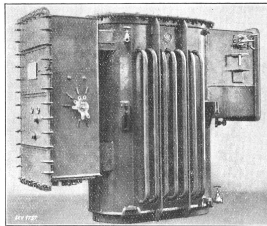
Fig. 10. Transformator 500 kVA, gekapselt, zum Einbau in Gruben, mit Netzschalter links und Erdungsschalter rechts.
