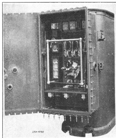
Fig. 11. Netzschalter des Transformators Fig. 10, geöffnet.
