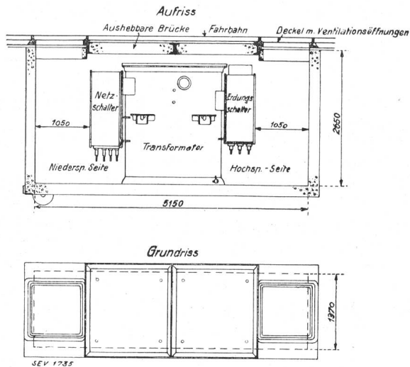
Fig. 8. Typische Transformatorgrube.
