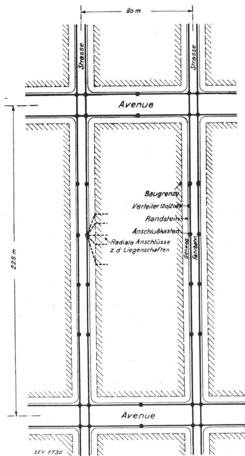
Fig. 3. Anordnung der Niederspannungsverteiler für einen typischen Strassenblock.
