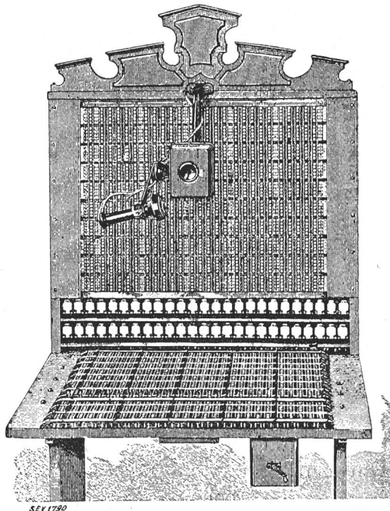
Fig. 4. Erste Umschaltvorrichtung.
