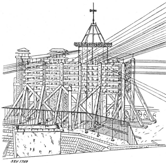
Fig. 3. Turm der ersten Zentralstation.
