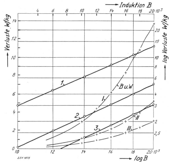
Fig. 1. Verlustkurven von Eisenblech. Analyse im doppellogarithmischen Masssystem. 1 \log B und \log W 50 Per/s. 2 \log B und \log W 25 Per/s. 3 \log B und \log W 16^{2/3} Per/s. I B und W 50 Per/s. II B und W 25 Per/s. III B und W 16^{2/3} Per/s.
