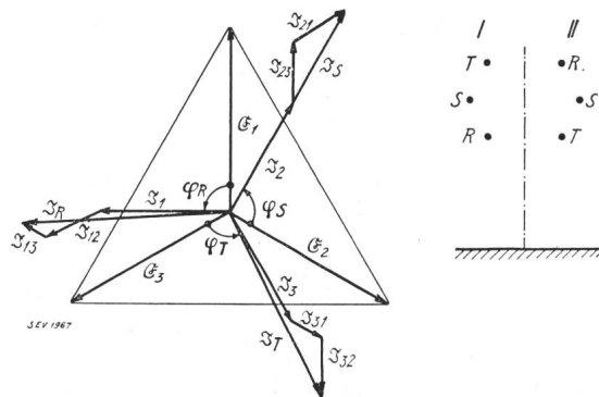
Fig. 6. Diagramm der leerlaufenden Leitung. Strang I. Rechts: Schema des Mastbildes. \mathcal{E}_1 \mathcal{E}_2 \mathcal{E}_3 Phasenspannungen. \mathcal{I}_R \mathcal{I}_S \mathcal{I}_T Leiterströme; diese setzen sich zusammen aus den Teilströmen \mathcal{I}_1, \mathcal{I}_{12} und \mathcal{I}_{13} etc. Phasenspannung und Leiterstrom sind gegeneinander verschoben, und zwar um mehr als 90^\circ in Phase R, um 90^\circ in Phase S und um weniger als 90^\circ in Phase T.
