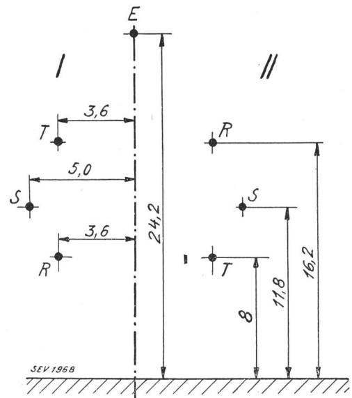
Fig. 7. Mastbild an Leitung Innertkirchen-Bickigen-Mühleberg. I Strang I. II Strang II. E Endseil. Alle Masse sind in m.
