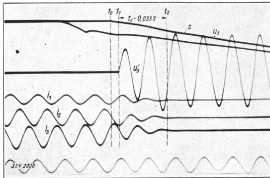
Fig. 2. s Oscillogramm einer lichtbogenfreien Abschaltung. Schaltbewegung. t_0 Anfang der Schaltbewegung. i_1 i_2 i_3 Ströme. u_3 wiederkehrende Spannung. t_1 Trennung der Schaltstücke. u_3 Spannungsabfall in der Flüssigkeit. t_2 Ende des Schaltvorgangs.
