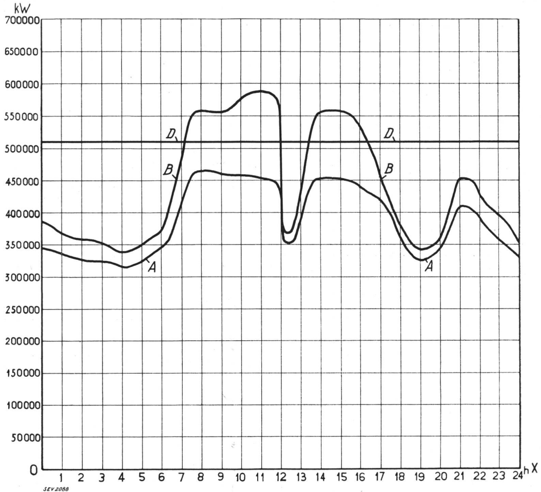
Verlauf der wirklichen Gesamtbelastungen am 13. Mai 1931. Diagramme journalier de la production totale le 13 mai 1931.
