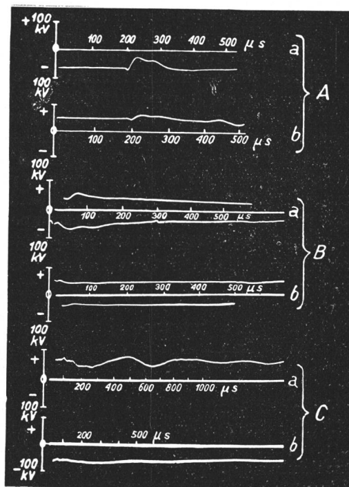
Fig. 15. Oscillogramme a : ligne B aboutissant à la station de mesure; l'oscillogramme indique la tension de l'onde réfléchie. Oscillogramme b : ligne A traversant la station de mesure; l'oscillogramme indique la tension de l'onde libre.
