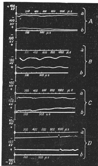
Fig. 16. Les deux lignes A B (Fig. 11) traversant la station de mesure.
