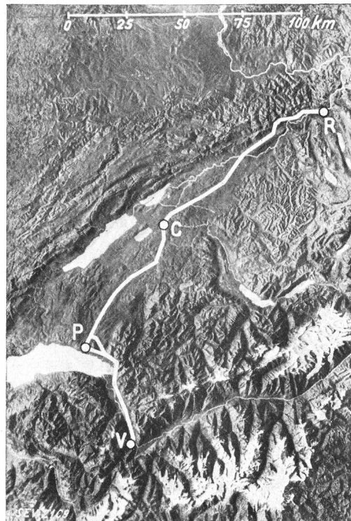
Fig. 4. Tracé de la ligne de transport 132 kV des Chemins de fer fédéraux.
