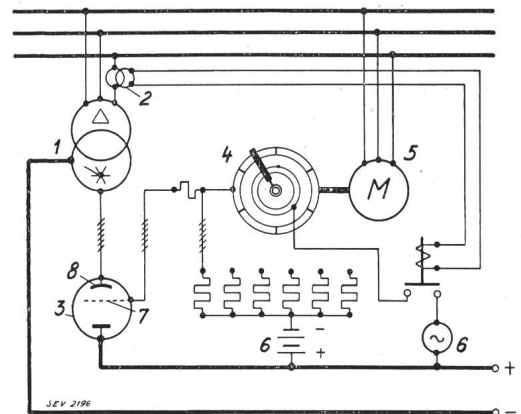
Fig. 5. Prinzipschema eines Gleichrichters mit Spannungsregulierung und Ueberstromschutz durch gesteuerte Gitter. 1 Transformator. 2 Stromwandler. 3 6-Phasengleichrichter. 4 Verteiler. 5 Motor zum Verteiler. 6 Steuerstromquelle. 7 Steuergitter. 8 Anode.
