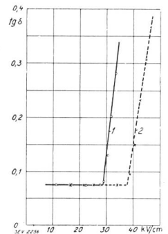
Fig. 7. tg \delta -Charakteristiken von Mikanitfolien zwischen Metallplatten. 1 vor der Pressung. 2 nach der Pressung.
