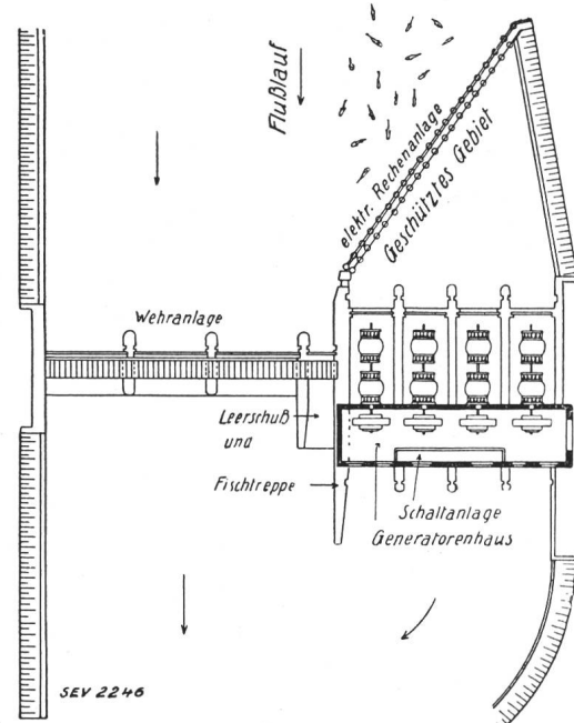
Fig. 2. Projekt eines Kraftwerkes mit eingebauter elektrischer Rechenanlage 2) .
