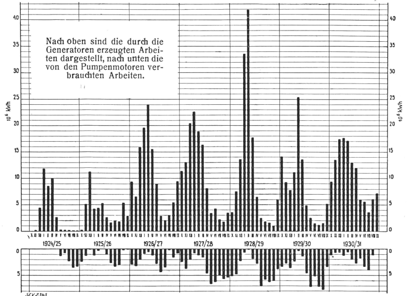
Fig. 30. Monatlich erzeugte Arbeit 1924 bis 1931.
