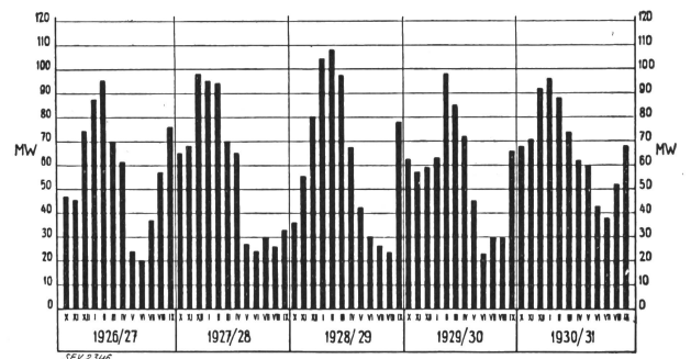
Fig. 31. Monatliche Höchstleistungen 1926 bis 1931.
