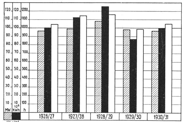
Fig. 32. Winterarbeit, Höchstleistung und Wintergebrauchsdauer 1926 bis 1931.
