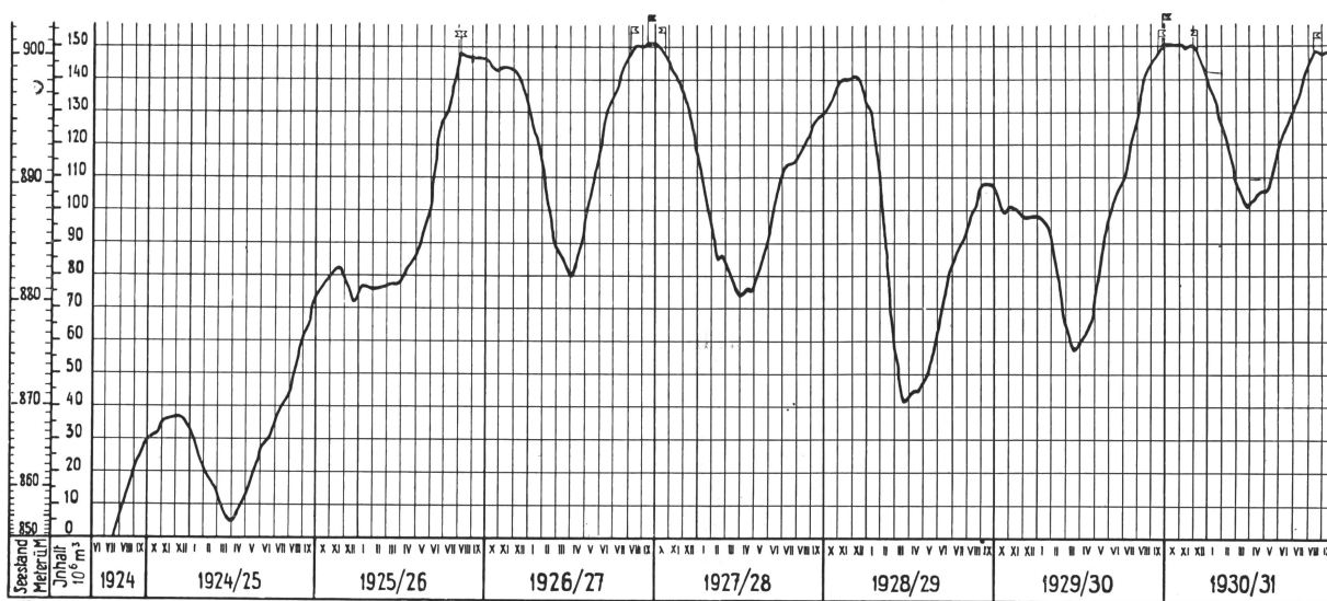
Fig. 33. Füllung des Stausees Innertal 1924 bis 1931. Kote 900 m \blacksquare Auffüllung \blacktriangle Kote 901 m Absenkung
