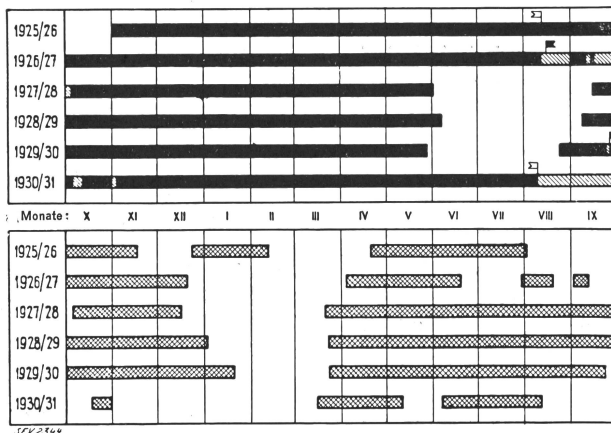
Fig. 29. Zeiten intensiven Turbinen- und Pumpenbetriebs 1925 bis 1931.
