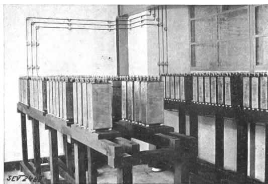
Fig. 3. Stationäre Pufferbatterie, Kapazität 132 Ah, 120 V.
