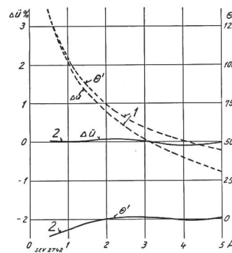
Fig. 37. Fehlerkurven ( \Delta u\% und \theta' ) des 400/5-A-Wandlers. D = 44 cm, H = 18 cm. Gewicht = 120 kg. Bürde = 0 bis 50 VA für \cos \varphi im Bereich von Fig. 39a. I Gewöhnlicher Wandler. II Präzisionswandler.
