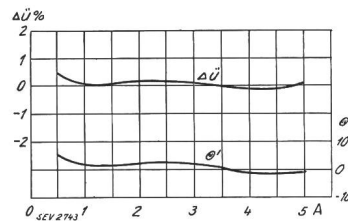
Fig. 38. Fehlerkurven ( \Delta u\% und \theta' ) des 200/5-A-Präzisionswandlers. D = 44 cm, H = 18 cm. Gewicht = 120 kg. Bürde = 0 bis 15 VA für \cos \varphi im Bereich von Fig. 39b
