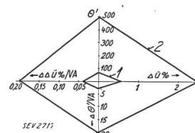
Fig. 11. Allgemeine Charakteristik eines 200/5-A-Wandlers. Bürde = 15 VA, \cos \varphi = 1 . 1 Legiertes Eisen. 2 Nickel-Eisen. D = 38 cm, H = 18 cm.
