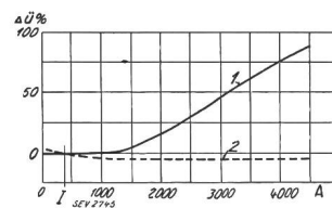
Fig. 39. 400/200/5-A-Wandler. Grenzen für Bürde und \cos \varphi .
