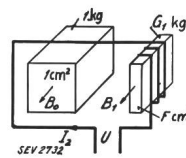
a Kernkombination mit proportionaler Beziehung zwischen Kraftflussverkettungen und Magnetisierungsstrom.
