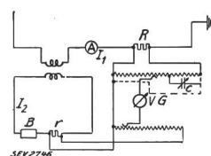
Fig. 42. Eichschaltung der Physikalisch-Technischen Reichsanstalt.
