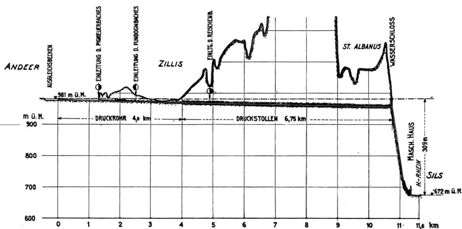
Fig. 2 (rechte Hälfte). Projekt für die Ausnutzung der Hinterrhein-Wasserkräfte. Gefällstufe Andeer-Sils. Masstab: Horizontal 1 : 375 000; Vertikal 1 : 37 500.
