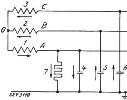
Fig. 8. Widerstandsdiagramm.
