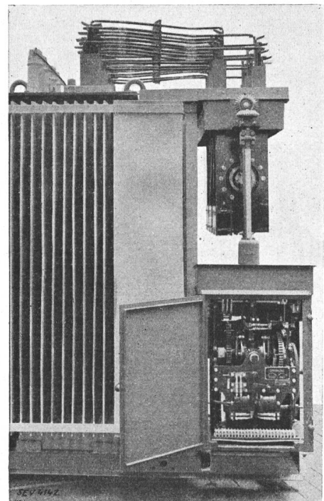
Fig. 7. Reguliertransformator mit Plattenstufenschalter (rechts oben).
