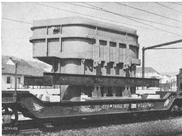
Fig. 22. Drehstromtransformator mit Regulierung für Freiluftaufstellung, 10 000 kVA, 148 000/6600 + 10 × 82,5 Volt, 50 Per./s, mit Trockenluftfüllung, Reglerschalter und Klemmen abgebaut, fertig auf Bahnwagen verladen.
