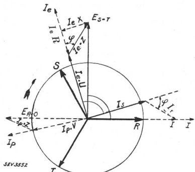
Fig. 13. Leistungsregler mit Stromdiagramm.
