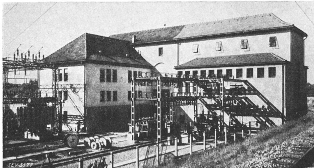
Fig. 18. Ansicht der Gebäulichkeiten des Unterwerkes mit den Drehstromfreiluftanlagen. Links: 43,5 kV-Anlage. Rechts: 8 kV-Anlage.
