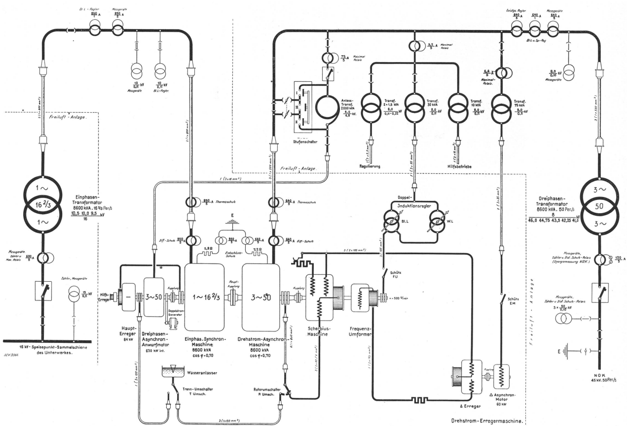
Fig. 3. Schaltungsschema der Umformergruppe.
