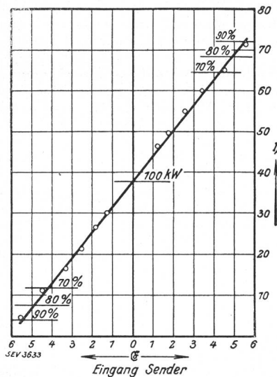
Fig. 2. Modulationskurve des Gross-Senders Wien.
