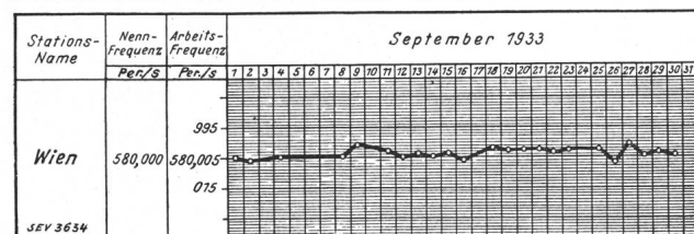
Fig. 3. Frequenzdiagramme des Gross-Senders Wien vom August und September 1933.
