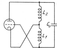
Fig. 6. Induktive Spannungsteilerschaltung.
