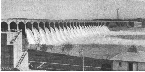
Fig. 1. Wilson-Damm mit Muscle Shoals-Kraftwerk jenseits des Tennessee-Flusses.
