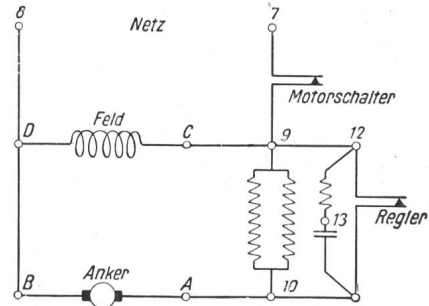
Fig. 6. Schaltung des Antriebs. (Maschine mit sechs-teiligem Stecker.)
