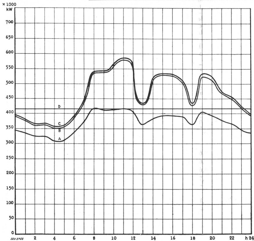
Diagramme de charge journalier du mercredi le 14 mars 1934.
