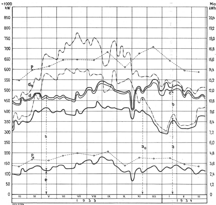
Diagramme annuel des puissances disponibles et utilisées, mars 1933 à mars 1934.
