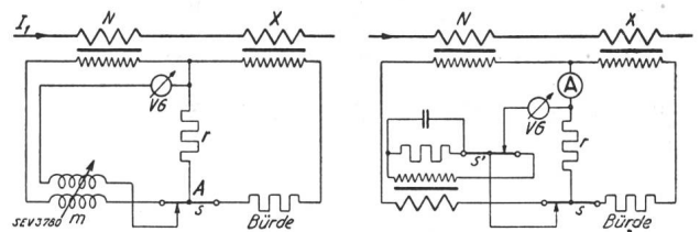
Fig. 3. Differentialenschaltung mit Kompensationskreis. Fig. 4. Ausgeführte Prüfungsschaltung.
