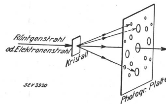
Interferenzen von Röntgenstrahlen oder Elektronenstrahlen an Kristallen.
