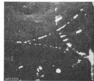
Fig. 15. Verwandlung eines \gamma -Quants in ein Elektronenpaar.
