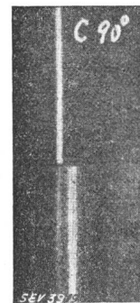
Spektralaufnahme der einfallenden (oben) und der gestreuten Strahlung (unten, nach rechts zunehmende Wellenlänge).
