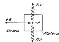
Fig. 18. Erzeugung von zwei Lichtquanten durch ein Positron (annihilation).
