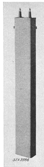
Fig. 22. Wellenglätter- Kondensator für 3000 Volt, 19 µ F.
