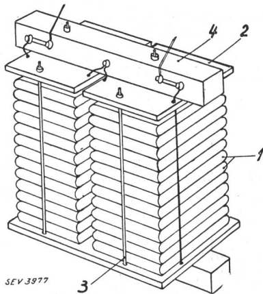
Fig. 11. Innenausbau eines Kondensators mit übereinander geschichteten Flachwickeln.
