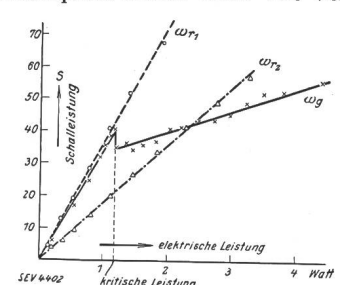
Fig. 2. Schalleistung in Abhängigkeit der elektrischen Leistung für normale ( \omega_1 ; \omega_2 ) und für «son rauque» ( \omega_0 ) Frequenzen.
