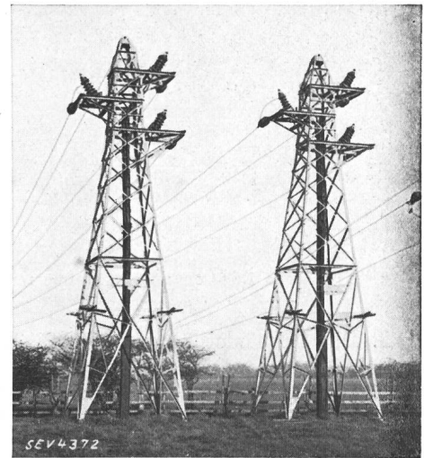
Fig. 5 b. 33 kV «Grid»-Sekundärleitungen. Kabel-Endmasten.
