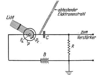
Fig. 3. Schaltung eines Mosaikelementes.
