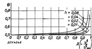
Fig. 6. Valeurs de \Theta dans le théorème des accroissements finis, appliqué au calcul de la courbe d'échauffement, pour \alpha = 1,25 .
