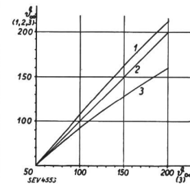
Fig. 11. Comparaison des diverses méthodes de calcul de la température finale. 1 \vartheta_\infty = \vartheta_n \frac{P_s}{P_n} 2 \vartheta_\infty = \vartheta_n \left(\frac{P_s}{P_n}\right) 3 \vartheta_\infty = \vartheta_n \left(\frac{P_s}{P_n}\right)^{0,8} \left[\frac{1 + a_b p_b \vartheta_\infty}{1 + a_b p_b \vartheta_n}\right]^\frac{1}{\alpha}
