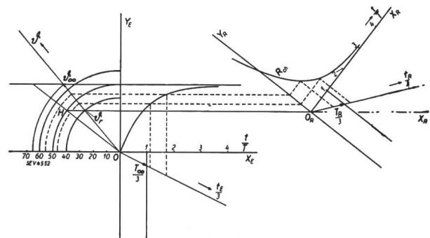
Fig. 10. Diagramme du service périodique pour un coefficient de transmission de la chaleur variable avec la température.
