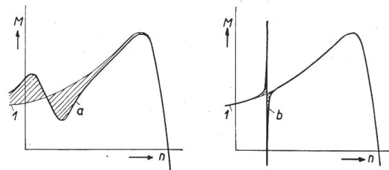
Fig. 8. Drehmoment-Drehzahl-Verlauf von Drehstrom-Käfiganker-Asynchronmotoren unter der Einwirkung von Oberfeldparasitär-momenten. (nach Kronldl). 1 Grundfeldmoment. a) Asynchrones Parasitär-moment. b) Synchrones Parasitär-moment. c) Vibrations-Parasitär-moment. (Zeitliche Mittelwerte des Drehmomentes.)
