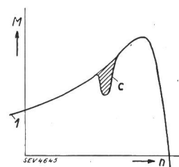
Fig. 8. Drehmoment-Drehzahl-Verlauf von Drehstrom-Käfiganker-Asynchronmotoren unter der Einwirkung von Oberfeldparasitär-momenten. (nach Kronldl). 1 Grundfeldmoment. a) Asynchrones Parasitär-moment. b) Synchrones Parasitär-moment. c) Vibrations-Parasitär-moment. (Zeitliche Mittelwerte des Drehmomentes.)
