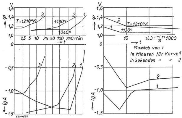
Fig. 1. Entaktivierungsvorgänge bei Emissionsbelastung. Fig. 2. Reaktivierungsvorgänge beim Glühen ohne Emission.
