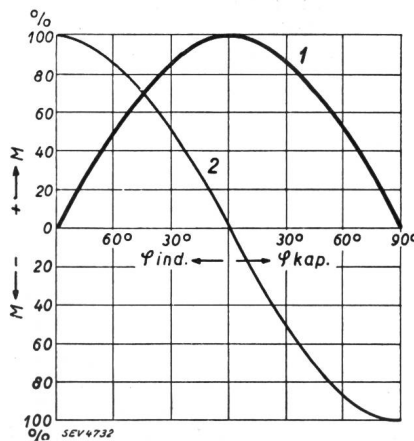
Fig. 6. Drehmoment des Wirkverbrauchzähler- (1) und Blindverbrauchzähler- (2) Zählersystems.
