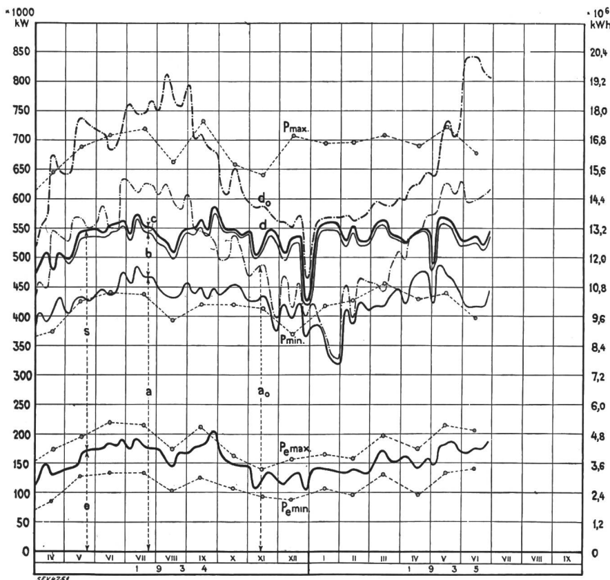
Diagramme annuel des puissances disponibles et utilisées, avril 1934 à juin 1935.
