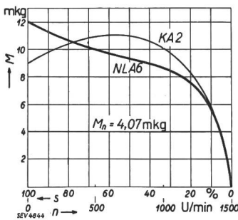
Fig. 34. 4 poliger Drehstrom-Asynchronmotor, 8 PS, mit nutzenlosem, radial geschichtetem Anker (NLA 6) nach Fig. 21 a und mit Käfiganker (KA 2) von gleichem Nennschlupf 50 \text{ Per./s}, U_1 \approx 330 \text{ V } \Upsilon Verlauf des Drehmomentes M mit der Drehzahl n . D_r = 199,2 \text{ mm } \varnothing, l_1 = 85 \text{ mm}.
