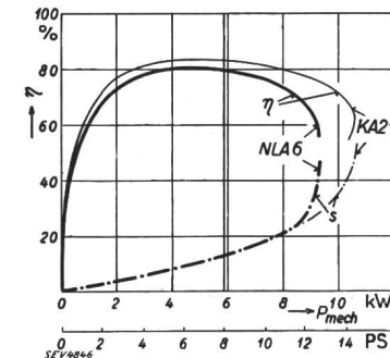
Fig. 36. Motor nach Fig. 34. Verlauf v. Wirkungsgrad \eta und Schlupf s mit der abgegebenen Leistung P_{\text{mech}} .
