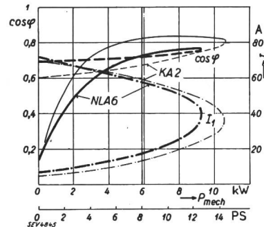
Fig. 35. Motor nach Fig. 34. Verlauf v. Leistungsfaktor \cos \varphi und Statorstrom I_1 , mit der abgegebenen Leistung P_{\text{mech}} .
