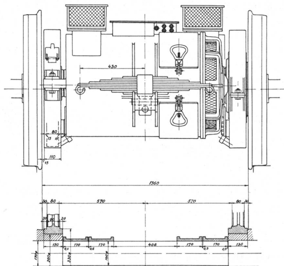
Fig. 3. Dessins de montage du moteur jumelé dans les 3 projections.
