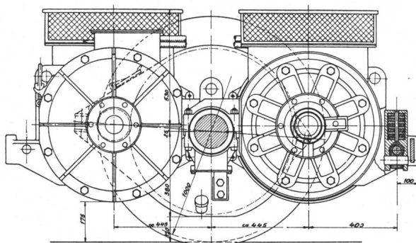
Fig. 2. Coupe transversale du moteur individuel.
