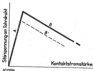
Fig. 1. Störspannung in Funktion der Kontaktstromstärke. A Löschkuntenzone — Totalunterbrechungen. B Lichtbogenzone — Schwankungen des Uebergangswiderstandes in endlichen Grenzen. B' Störkennlinie bei schwächerer Riffelung, d. h. kleineren Distanzierungen am Wanderkontakt.
