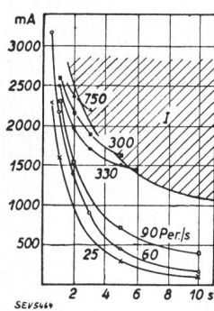
Fig. 1. Minimalströme in mA für verschiedene Frequenzen in Abhängigkeit von der Durchflusszeit in s. I Gebiet der Hyperpyrexie.
