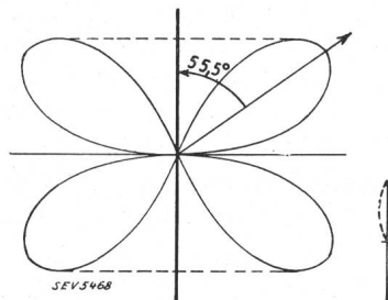
Fig. 3. Strahlungscharakteristik einer freien, in der zweiten Harmonischen schwingenden Antenne.
