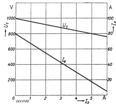
Fig. 5. pour U_2 = 90 kV, couplage 1000 V.
