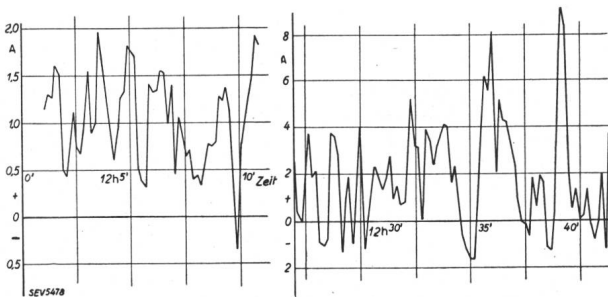
Fig. 4A. Strom im 25 mm-Rohr. Strom im 40 mm-Rohr.
