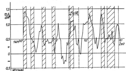
Fig. 6. Schwankungen des aus der Sonde am 25 mm-Rohr strahlenden Stromes, in Abhängigkeit vom Verkehr der Stadtbahnzüge.
