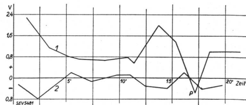
Fig. 7. Mittlere Spannungsunterschiede zwischen dem 25 mm-Rohr und dem 40 mm-Rohr.
