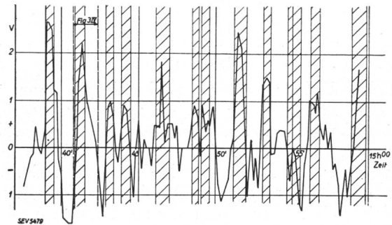
Fig. 5. Schwankungen der Spannung zwischen dem 25 mm-Rohr und dem 40 mm-Rohr in Abhängigkeit vom Verkehr der Stadtbahnzüge. Die schraffierten Teile geben die Anfahrtsperioden der Züge an.
