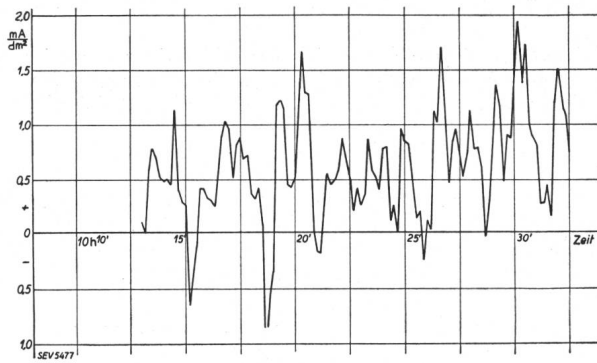
Fig. 4. Sondennmessungen am Rohr von 25 mm \varnothing .
