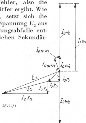
Fig. 1. Normales Stromwandlerdiagramm.
