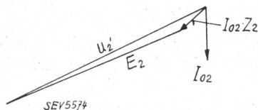
Fig. 2. Stromwandlerdiagramm bei sekundärseitiger Speisung und offener Primärwicklung.
