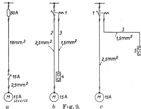
Fig. 9. a Installation bei Verwendung von Hand-Motorschalters. b Billigere Installation bei Verwendung von ferngesteuertem Motorschutzschalter. c Bedienung des Motors mit Fernsteuerung von geeignetster Stelle aus. 1 Ferngesteuerter Motorschutzschalter. 2 Motorleitung 2,5 mm 2 . 3 Steuerleitung 1,5 mm 2 . 4 Bedienungsdrukknöpfe. 5 Druckknöpfe an geeignetster Bedienungsstelle.
