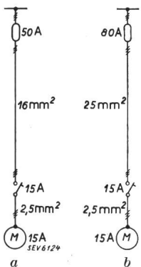
Fig. 8. Selektivität zwischen Querschnittsicherung und Selbstschalter. a Bei Verwendung von Selbstschalter mit thermischer Ueberstrom- und elektromagnetischer Schnellauslösung muss die Querschnitt-Sicherung für 50 A bemessen sein. b Bei Verwendung von Selbstschalter mit rein thermischer Ueberstromauslösung muss die Querschnitt-Sicherung für 80 A bemessen sein.
