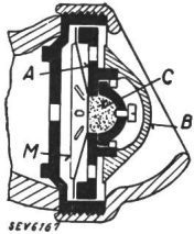
Fig. 3. USA-Mikrophon.
