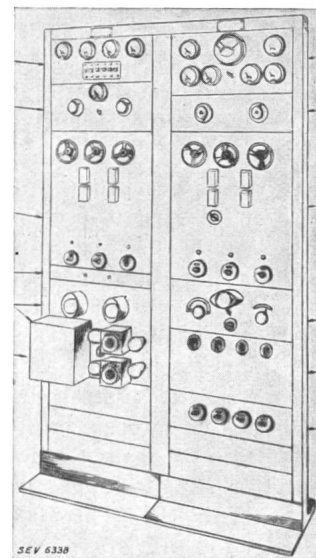
Fig. 22. Equipement à micro-ondes de la station de Lympne. 1 instruments de mesure de l'amplificateur. 2 réglage de la modulation. 3 réglage de l'émetteur à micro-ondes. 4 raccordement de contrôle. 5 amplificateur à basse fréquence (émetteur). 6 amplificateur à basse fréquence (récepteur). 7 instruments de mesure pour le contrôle des micro-ondes. 8 démodulateur. 9 réglage du récepteur à micro-ondes. 10 oscillateur à 500 kHz. 11 raccordement de l'amplificateur au réseau. 12 interrupteur de réseau.
