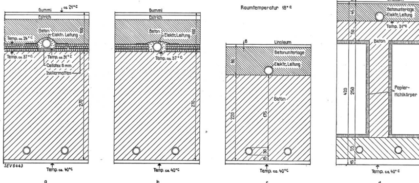
Fig. 1. Verschiedene Bodenbauarten mit Deckenheizung.
