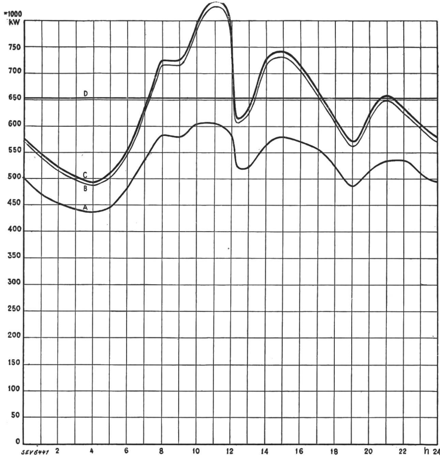
Diagramme de charge journalier du mercredi 18 août 1937.
