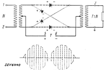
Fig. 1. Modulationsvorgang im Ringmodulator.
