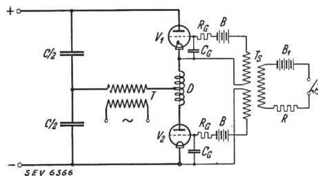
Fig. 6. Steuerkreisschaltung.
