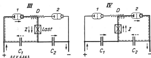
Fig. 3. Einfachschtung und Doppelschtung.
