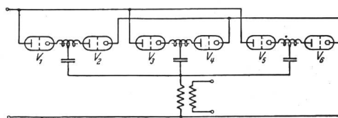
Fig. 5. Speicherwechselrichter für hohe Frequenzen.
