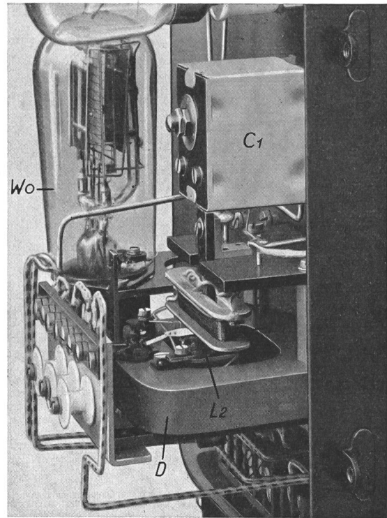
Fig. 4. Messwertverstärker.
