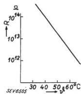
Fig. 3. Mit steigender Temperatur T sinkt der elektrische Widerstand R beim Schellack.
