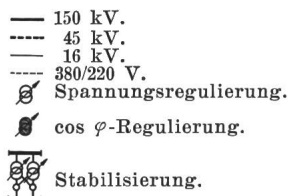
Fig. 4. Super-Netz mit Spannungsregulierung.
